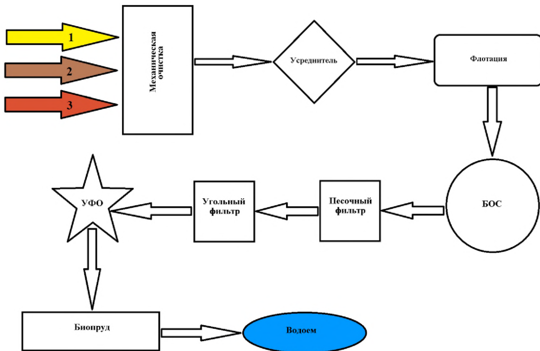
Рис. 1. Схема очистки сточных вод
