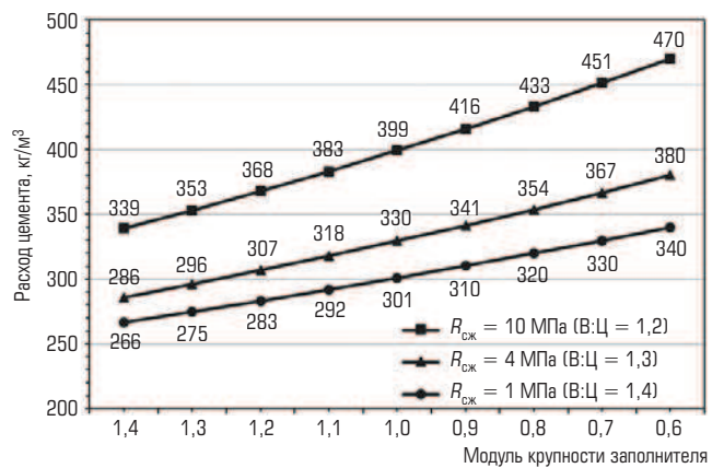
Рис. 1. Расход цемента на 1 м 3 закладочной смеси в зависимости от модуля крупности заполнителя и требуемой прочности.
