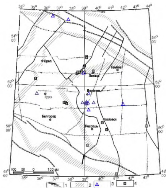
Рис. 1. Пространственное положение промышленных карьеров, в которых производятся наиболее мощные взрывы. Обозначения: 1 – тектонические нарушения разных рангов; 2 – зоны сочленения геологических блоков; 3 – пункты сейсмологического наблюдения региональной сети; 4 – промышленные карьеры
