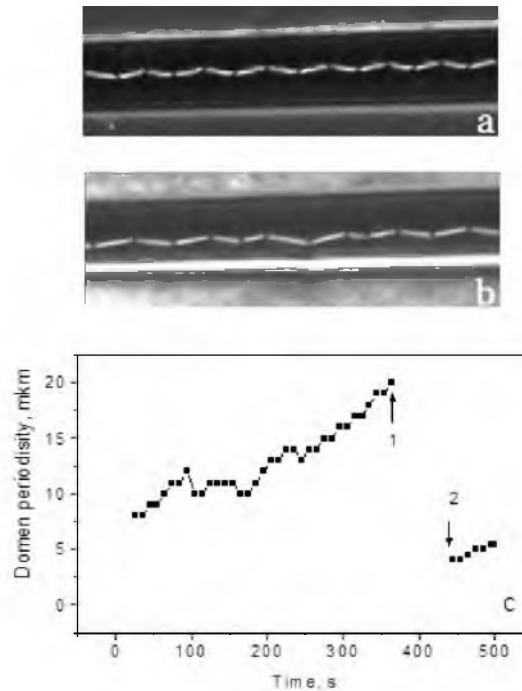
Рис. 8. Домешная текстура в «толстом» слое нематика при возрастании концентрации ДМ. а – исходная доменная текстура. б – время действия пара ДМ 200 секунд. с – зависимость шага расположения доменов от времени действия пара ДМ. Ячейка с открытой поверхностью нематика 5СВ. Напряжение – 6,5 В. Частота – 50 кГц.
