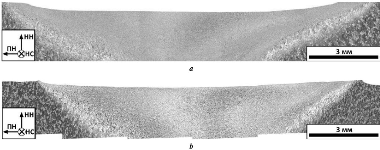
Рис. 2. Панорамные EBSD-карты, иллюстрирующие макроструктуру поперечного сечения сварных соединений: a – низкотемпературный режим; b – высокотемпературный режим. Система координат: НС – направление сварки; ПН – поперечное направление; НН – направление нормали к плоскости свариваемых листов
