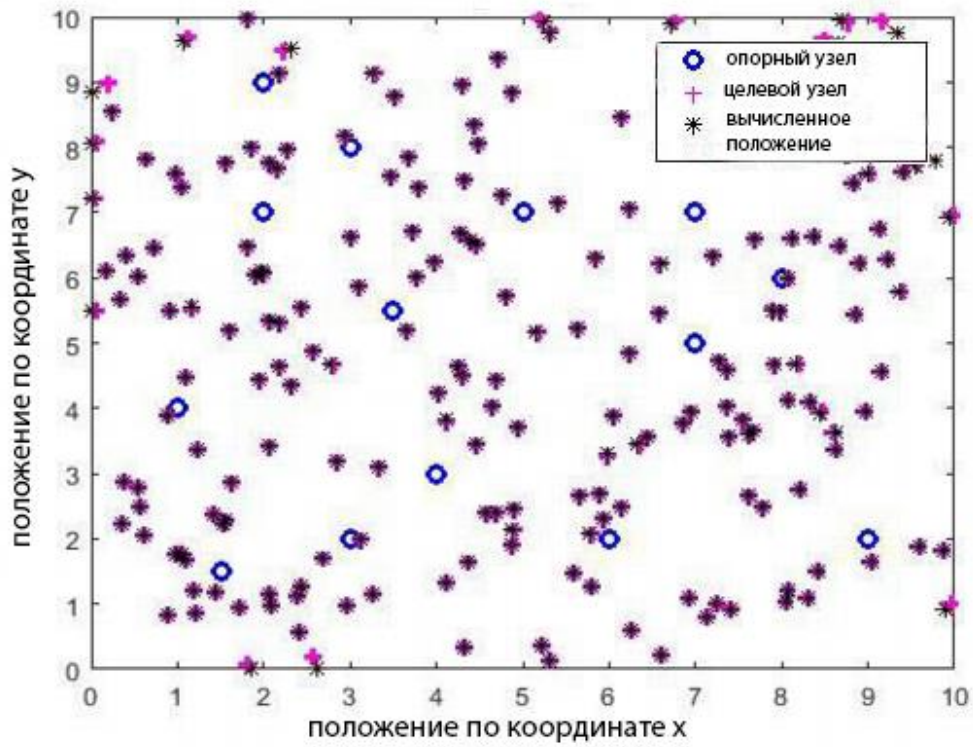
Рис. 7. Локализация с использованием TDoA, при n=200 Fig. 7. Localization using TDoA, at n=200
