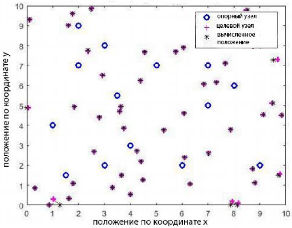
Рис. 6. Локализация с использованием TDoA, при n=50 Fig. 6. Localization using TDoA, at n=50
